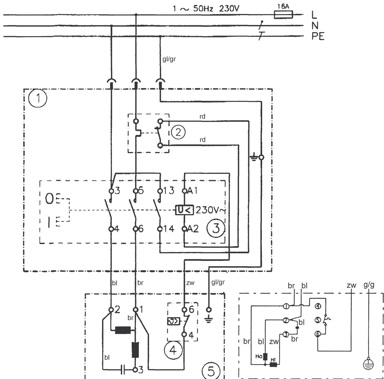
Klem-aansluitschema in motor
