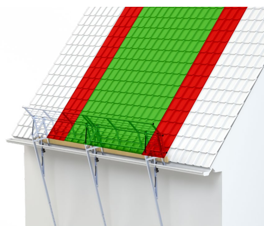
toegestaan werkgebied
