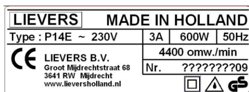
Abb. 1: Muster Typenschild P14E
