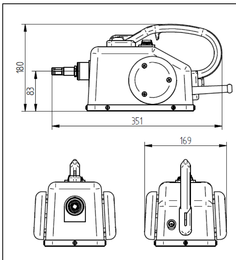
Abb. 4 Abmessungen der P14E Antriebseinheit in mm
